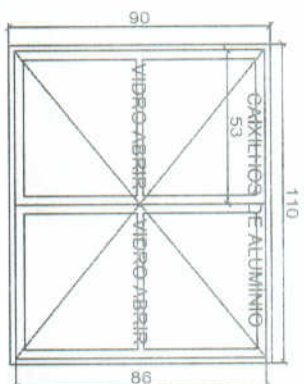
JANELA 1,10mx0,90m VIDRO ABRIR 3 UNIDADES MODELO 11
