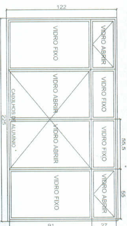
JANELA 2,25mx1,22m 1 UNIDADE MODELO 10
