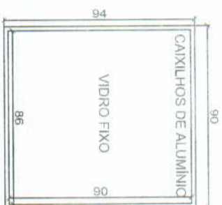
JANELA 0,90mx0,94m VIDRO FIXO 1 UNIDADE MODELO 03
