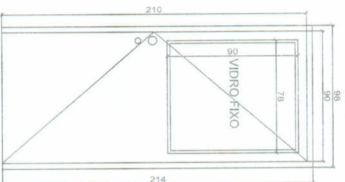
PORTA 0,90mx2,10m COM VIDRO FIXO 5 UNIDADES MODELO 09
