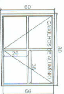
JANELA MAXIMAR 0,80mx0,60m 2 UNIDADES MODELO 08
